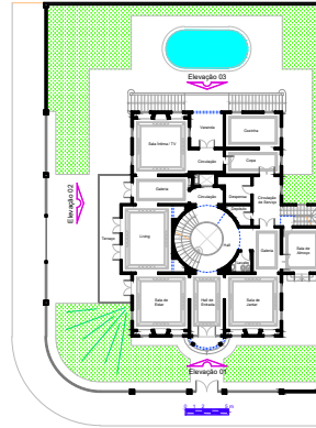
Térreo A = 302,17 m 2
