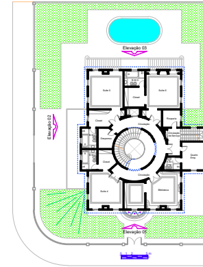
1º Andar A = 295,18 m 2
