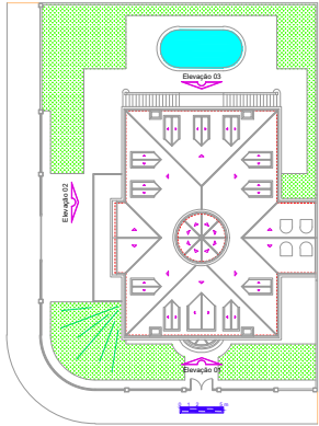
Implantação e Cobertura
