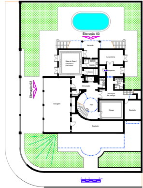
Subsolo A = 312,79 m 2
