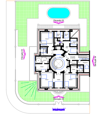
2º Andar A = 266,64 m 2
