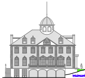
Elevação 02
